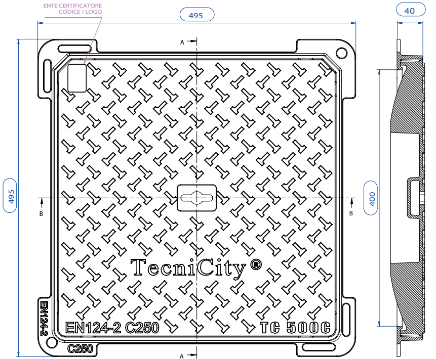
SEZIONE A-A
