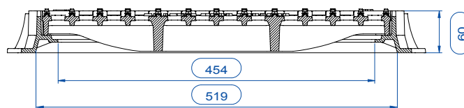
SEZIONE B-B
