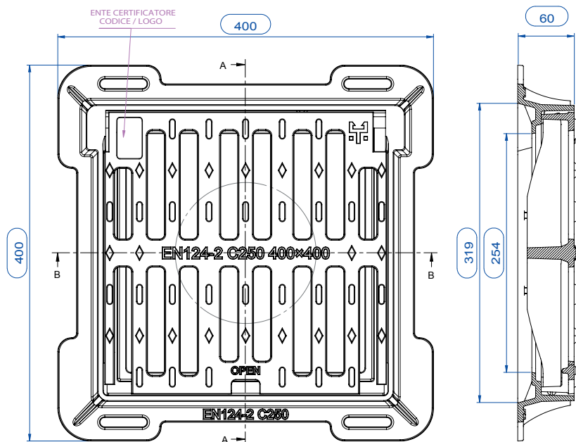
SEZIONE A-A
