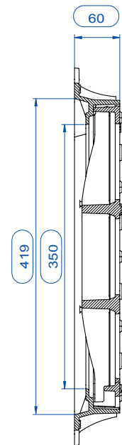
SEZIONE A-A
