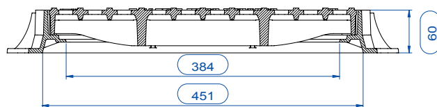
SEZIONE B-B
