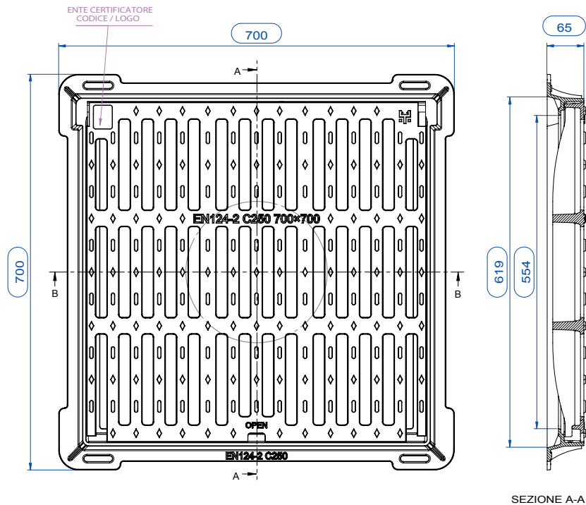
SEZIONE A-A
