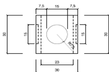
vista frontale - scala 1:10
