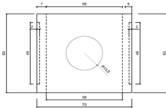
Pianta - scala 1:10
