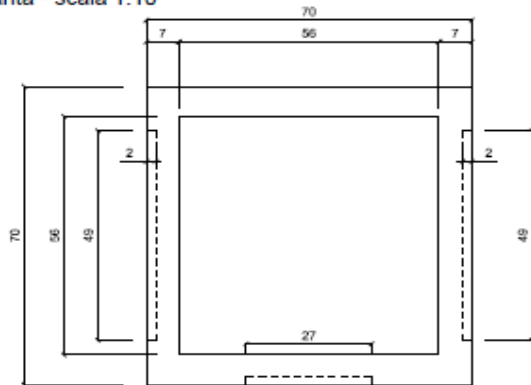
Pianta - scala 1:10
