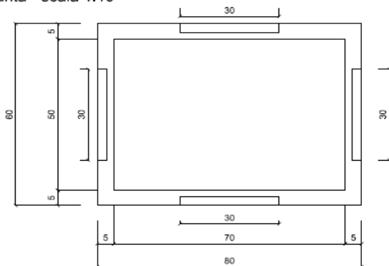
Planta - scala 1:10
