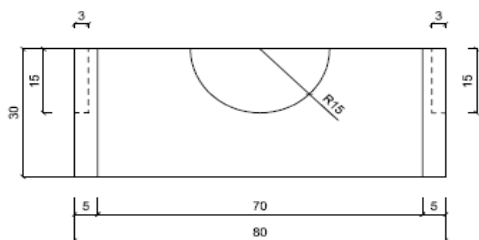
Planta - scala 1:10
