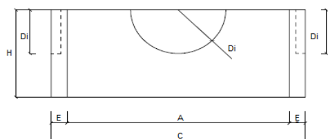
Pianta - scala 1:10
