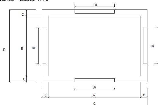
Pianta - scala 1:10
