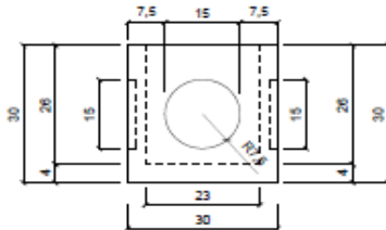
vista frontale - scala 1:10
