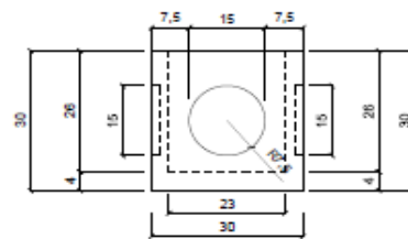
vista laterale - scala 1:10
