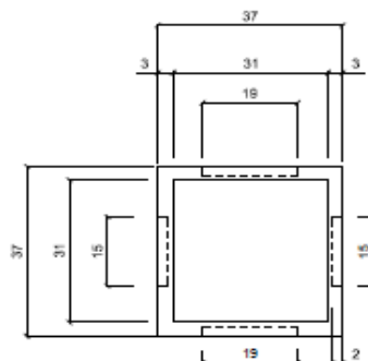
Pianta - scala 1:10
