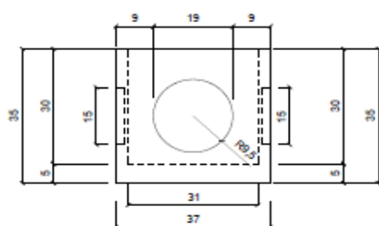
Pianta - scala 1:10
