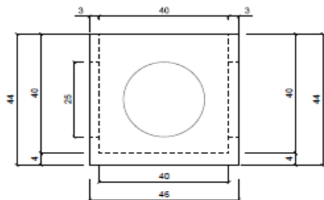
Pianta - scala 1:10
