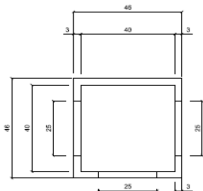
Pianta - scala 1:10
