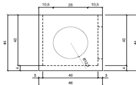
vista laterale - scala 1:10
