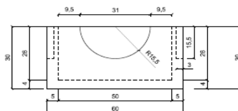
vista laterale - scala 1:10
