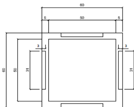
Pianta - scala 1:10
