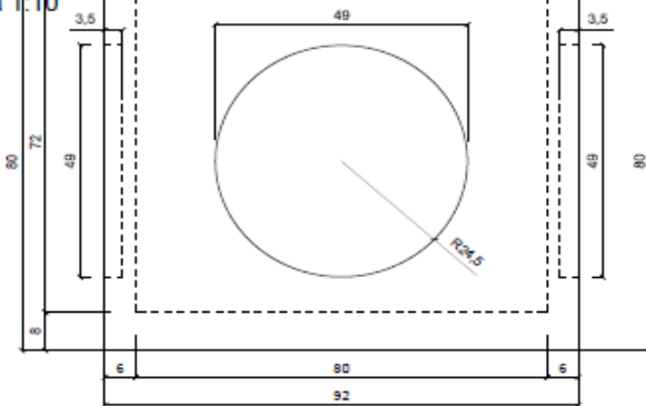
Pianta scala 1:10
