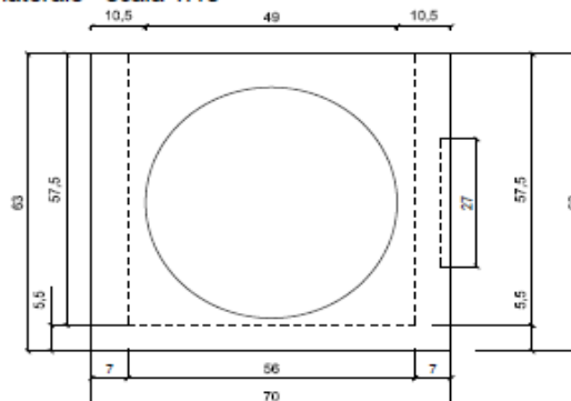
vista laterale - scala 1:10
