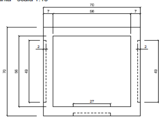
Pianta - scala 1:10
